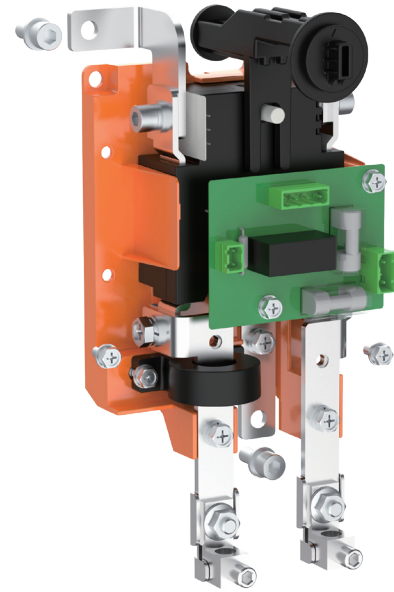
Generator Module
